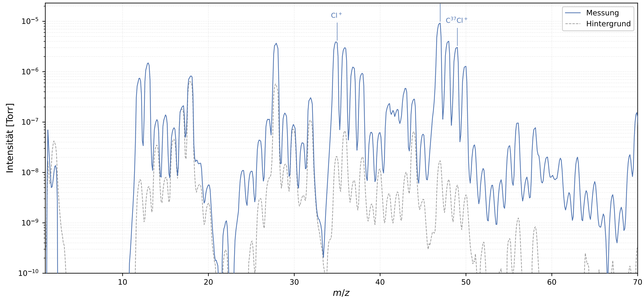
Chloroform ( \text{CHCl}_3 , M = 119 ) — Messung und Hintergrund (logarithmisch)
